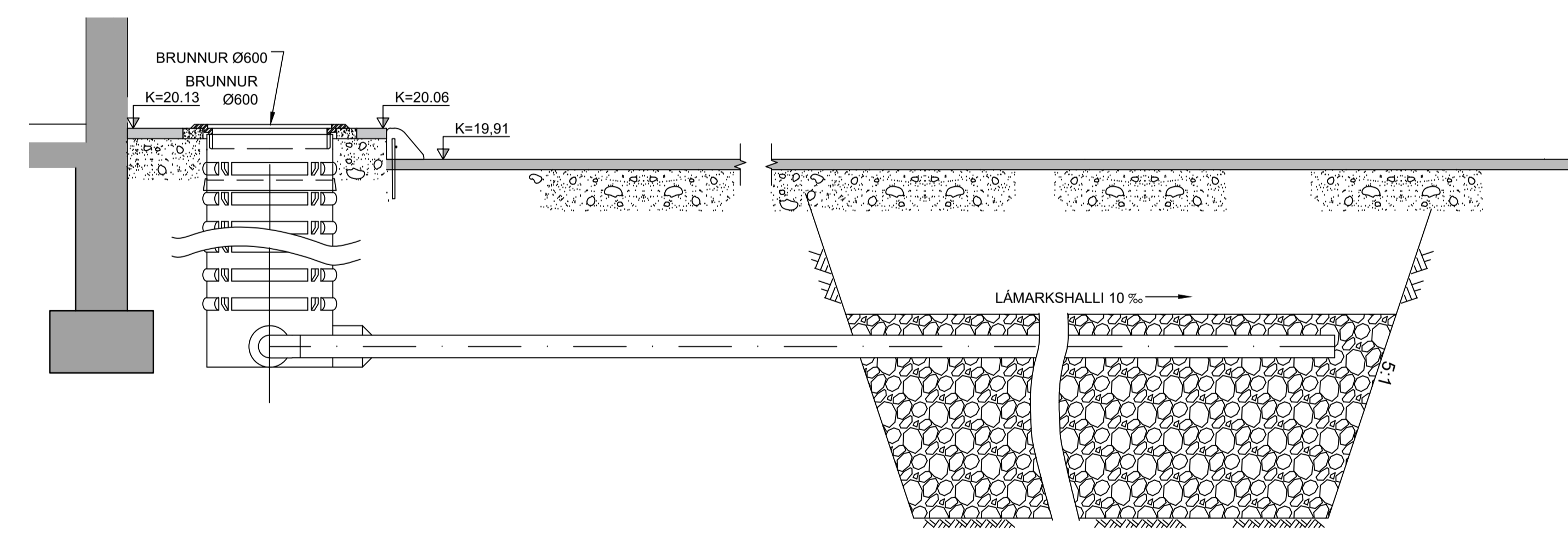
06 SNID 1011 1:20
