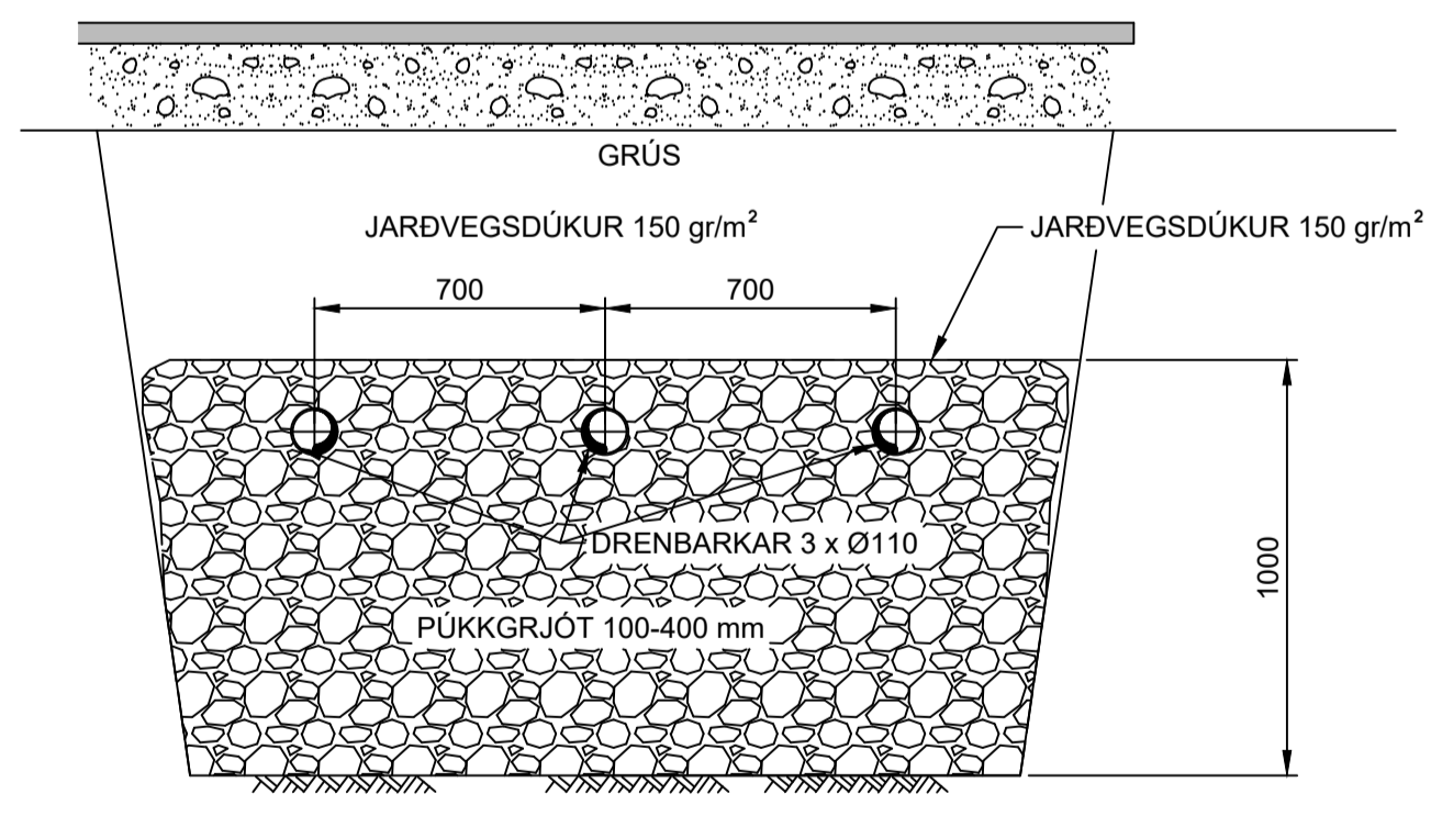
ÞVERSNIÐ Í PÚKK 1:20
