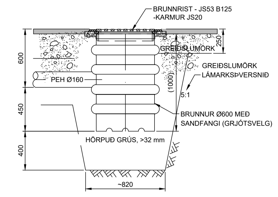
FRÁGANGUR BRUNNA 1:20
