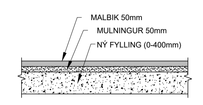
UPPBYGGING MALBIKAÐS PLANS 1:20
