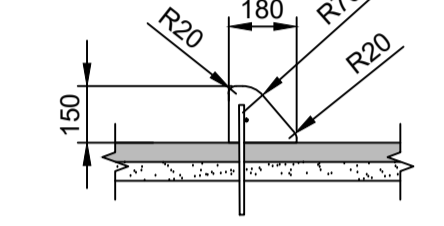
KANTSTEINN 1:20
