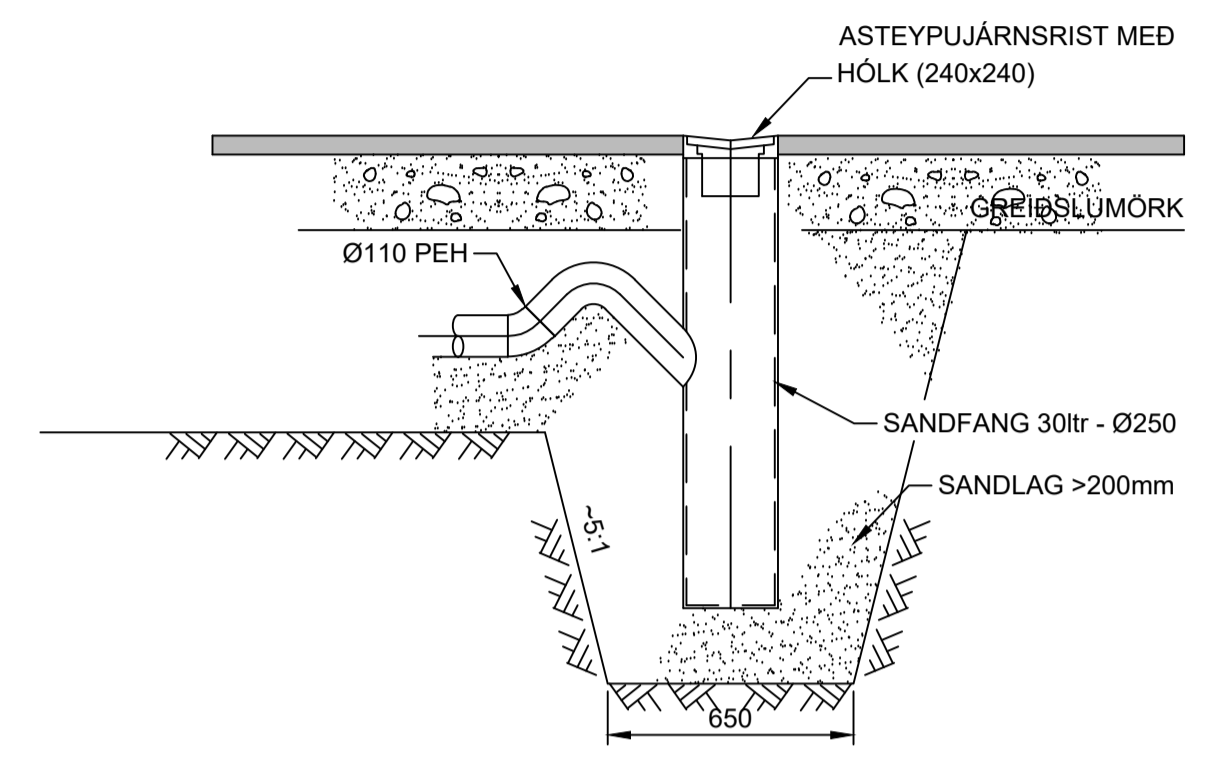
FRÁGANGUR NIÐURFALLA 1:20
